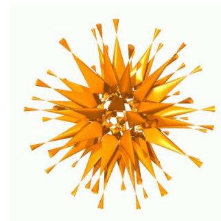
DECIC
