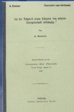
Äquivalenzformel E=mc^2
