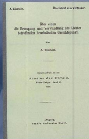
Photoeffekt: Nobelpreis 1921
